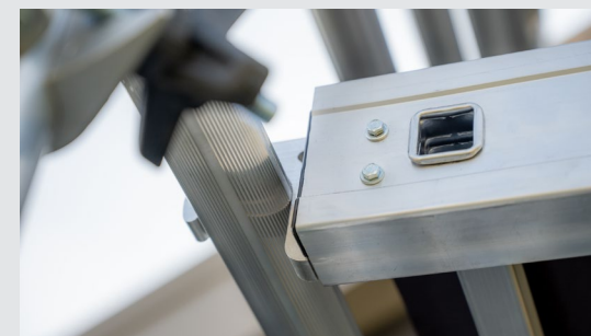
Asymmetrische platformhaken voor doorbouwen
