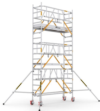
Ook beschikbaar als smalle steiger
